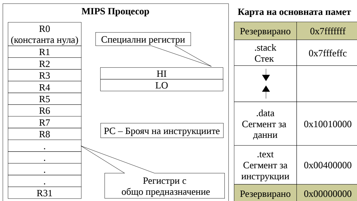
Фиг. 4. Разпределение на регистрите и паметта в MIPS
