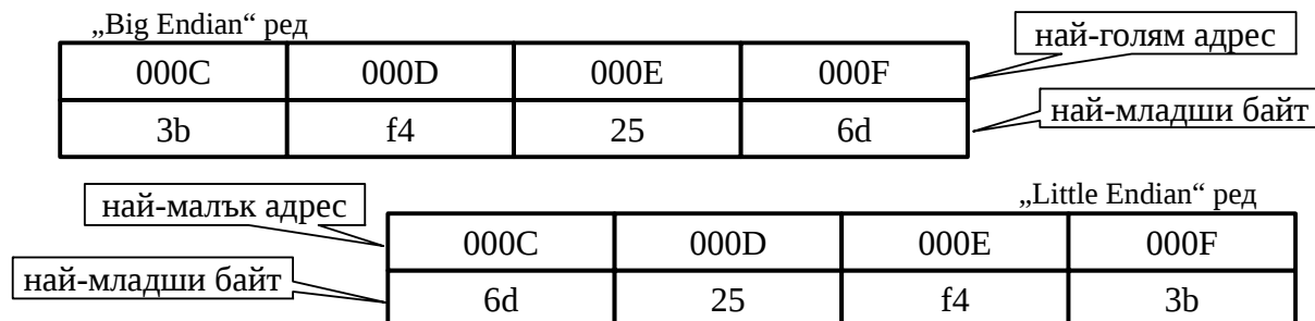
Фиг. 3. Подреждане на данните в паметта
